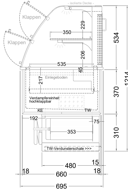
(Seitenansicht)
