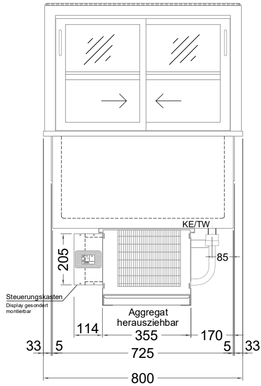
(Grundriss)
